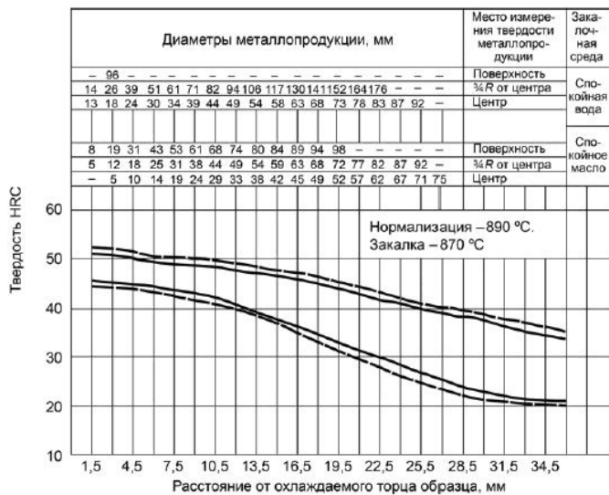
Рисунок А.10 - Сталь марки 27ХГР
