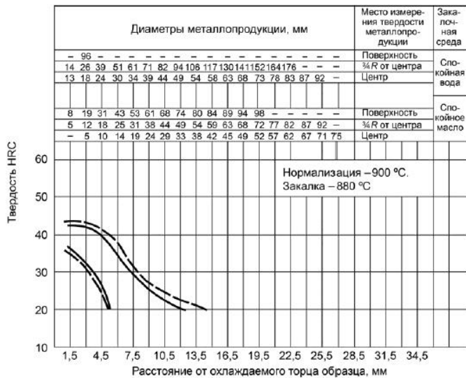
Рисунок А.1 - Сталь марки 15X
