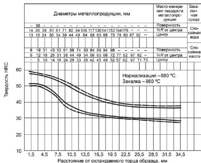
Рисунок А.14 - Сталь марки 40ХФА
