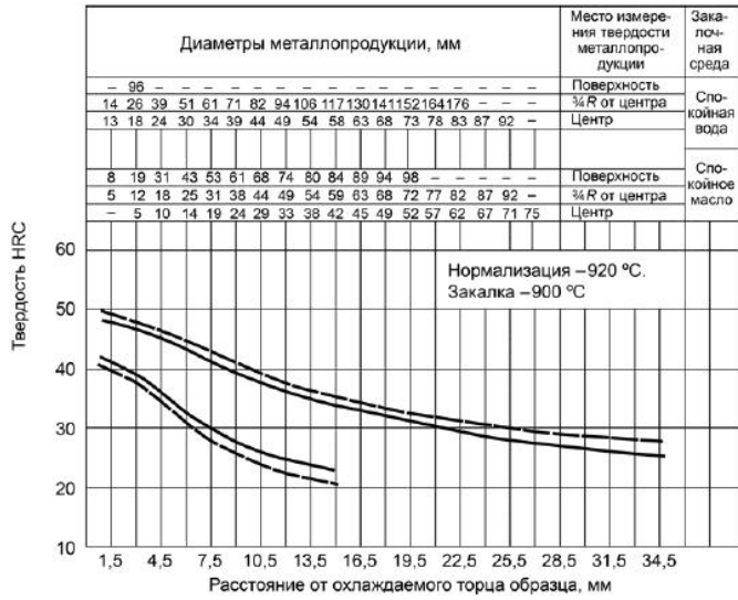
Рисунок А.7 - Сталь марки 18ХГТ
