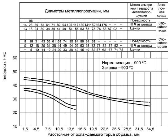
Рисунок А.9 - Сталь марки 20ХГР
