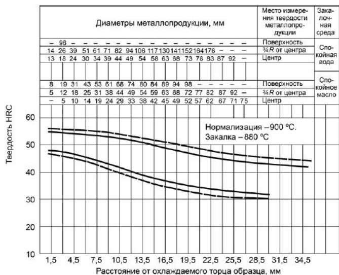
Рисунок А.13 - Сталь марки 38ХС
